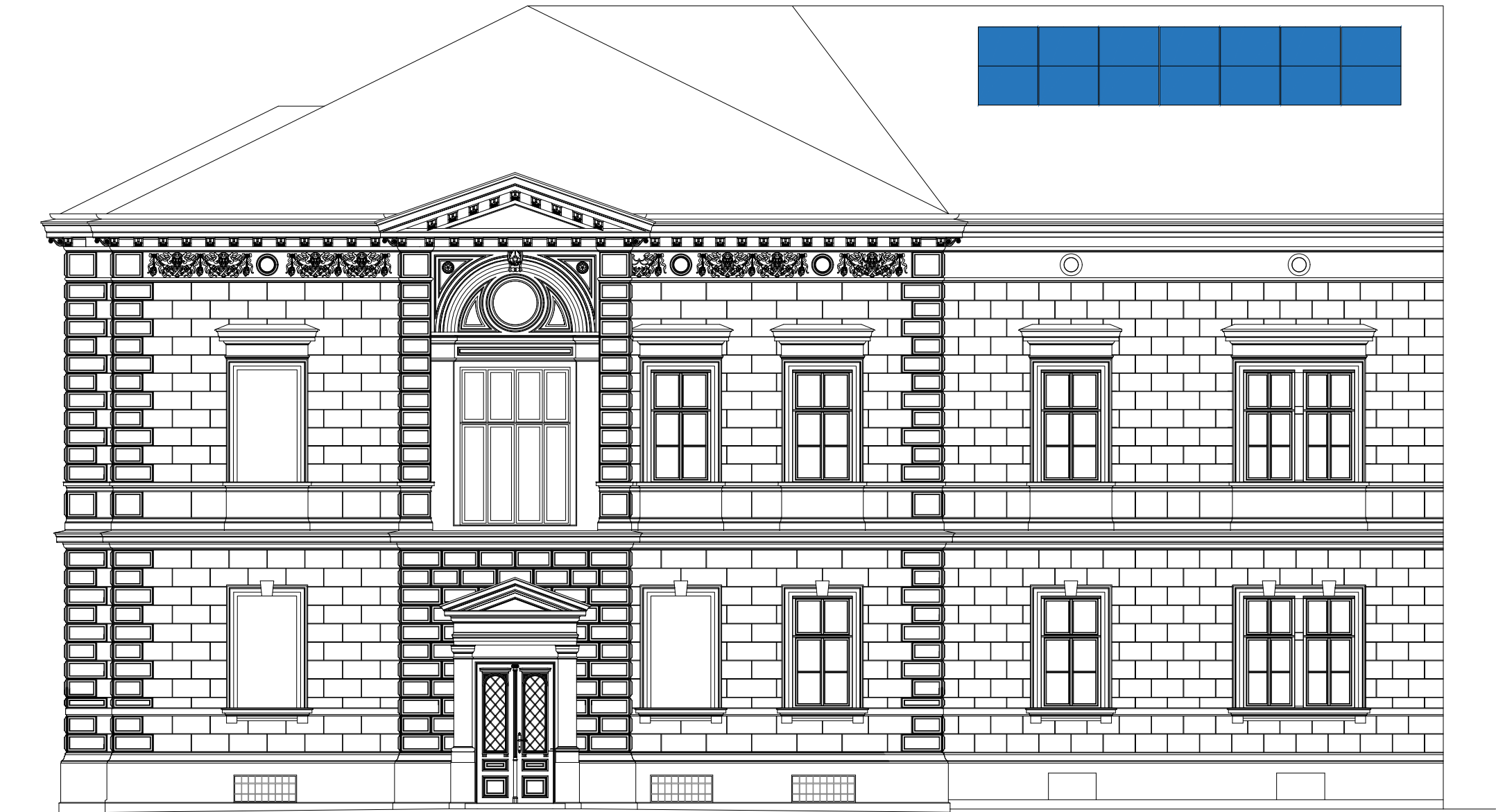
ZAPADNO PROČELJE
